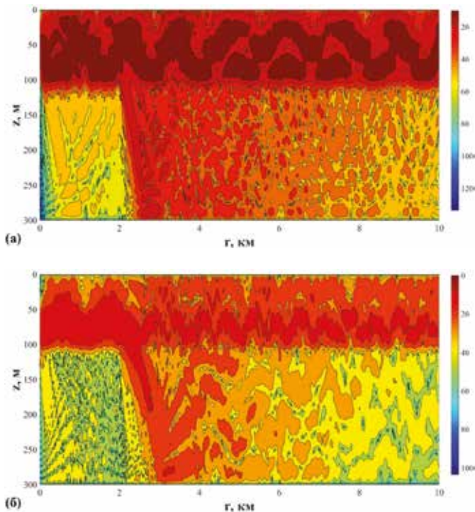
Рис. 7. Зависимость потерь на распространение TL от пространственных координат для Модели I и тонального сигнала с частотой 100 Гц. Рис.6 (а) соответствует гауссову пучку с p = 0.07 и z_0 = 55 м, что соответствует «пятну проходимости» на рис. 6(б). Рис. 6(б) соответствует гауссову пучку, преимущественно распространяющемуся в придонном звуковом канале
