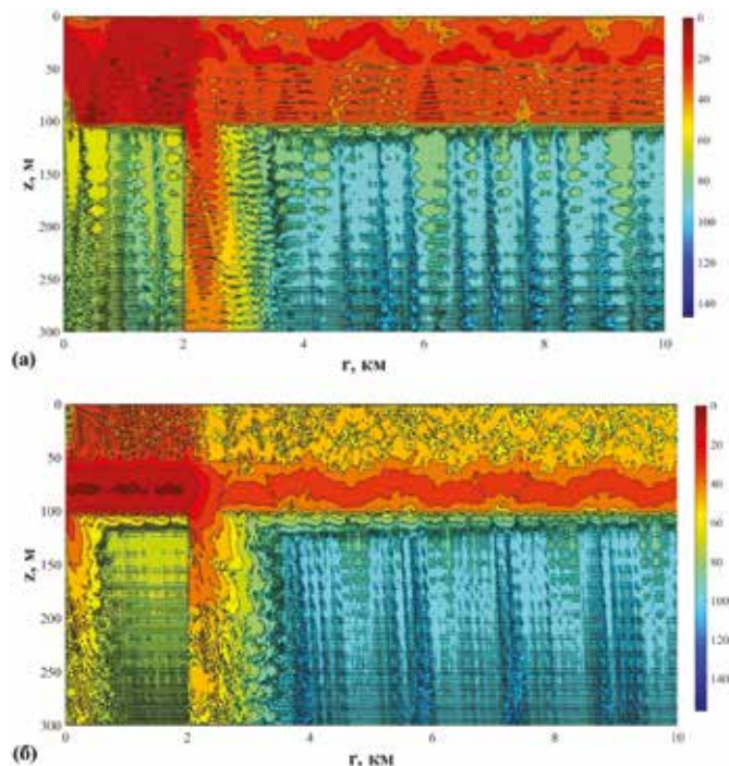
Рис. 9. Зависимость потерь на распространение TL от пространственных координат для Модели 1 и тонального сигнала с частотой 400 Гц. Панель (а) соответствует гауссову пучку с p = 0.07 и z_0 = 30 м, что соответствует «пятну проходимости» на рис. 8(б). Панель (б) соответствует гауссову пучку, преимущественно распространяющемуся в придонном звуковом канале
