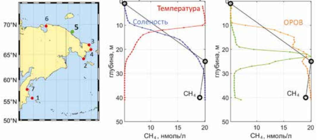
Рис. 6. Станция № 5 около пролива Лонга на шельфе Чукотского моря, 13 августа 2013 г.: вертикальный профиль распределения концентраций метана, нмоль/л; относительный ход температуры, °С; солености, S ‰; концентрация хл-а и ОРОВ в водной толще.
