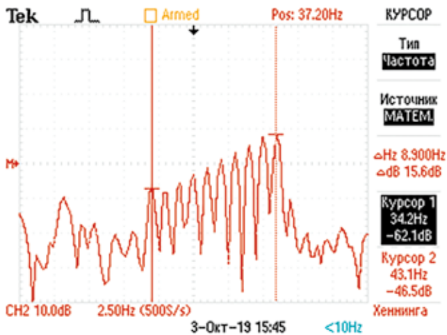
Рис. 6. Спектр полигармонического сигнала на контрольном гидрофоне
