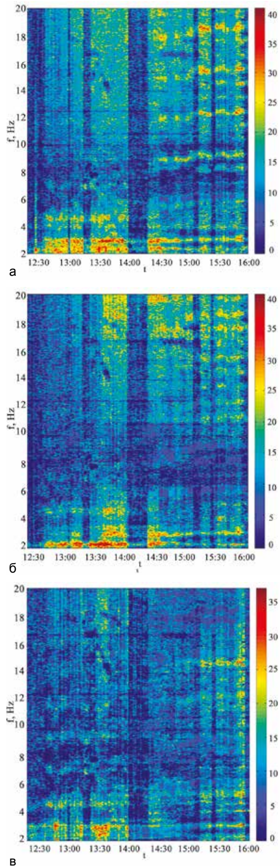
Рис. 10. Сонограммы для оценки помехоустойчивости КП, приемные модули: ПМ-1 (а); ПМ-2 (б); ПМ-3 (в)
