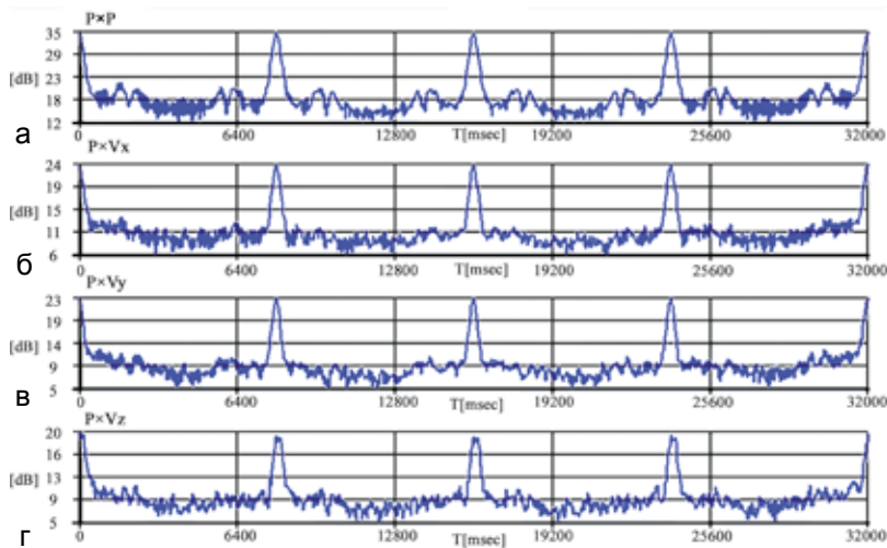
Рис. 15. Функции автокорреляции и взаимной корреляции между сигналом P(t) и сигналами в каналах P(t) , V_x(t) , V_y(t) , V_z(t) ; ПМ-1(а); ПМ-2(б); ПМ-3 (в); ПМ-4 (г); V_z(t) , приемный модуль ПМ-1, масштаб логарифмический
