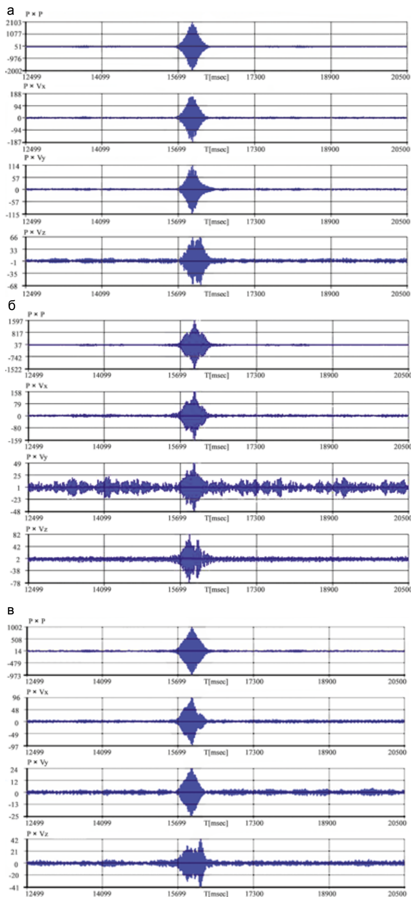
Рис. 14. Функции автокорреляции и взаимной корреляции между сигналом P(t) и сигналами в каналах P(t) , V_x(t) , V_y(t) , V_z(t) ; приемные модули: ПМ-1 (а); ПМ-2 (б); ПМ-3 (в)
