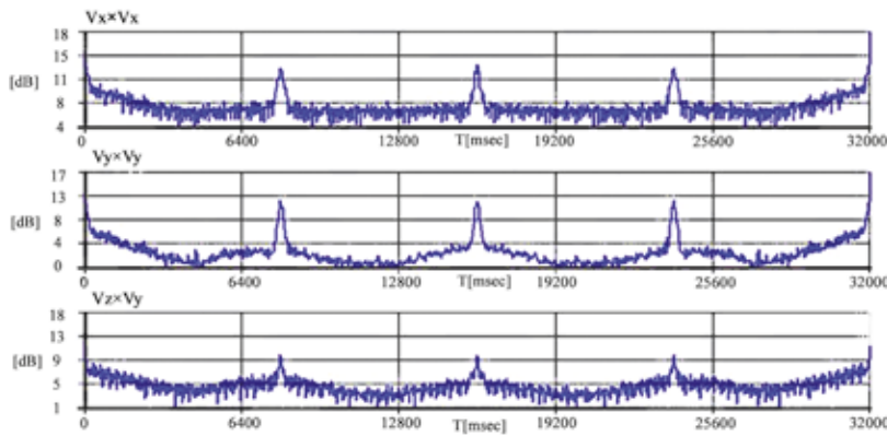
Рис. 16. Функции автокорреляции в векторных каналах V_x(t) , V_y(t) , V_z(t) , приемный модуль ПМ-1, масштаб логарифмический
