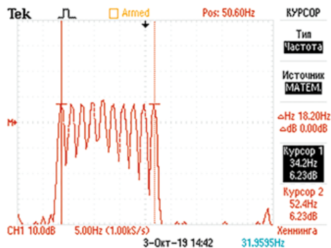
Рис. 3. Спектр полигармонического сигнала в диапазоне частот 34–43 Гц
