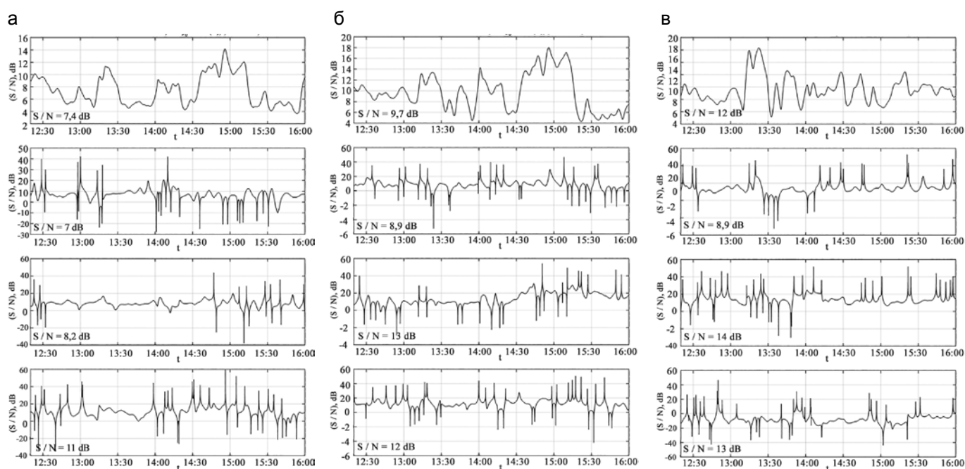
Рис. 11. Проходные характеристики для отношения (S/N) в каналах КП, приемные модули: ПМ-1 (а); ПМ-2 (б); ПМ-3 (в), частотный диапазон 16–20 Гц, время усреднения 50 с
