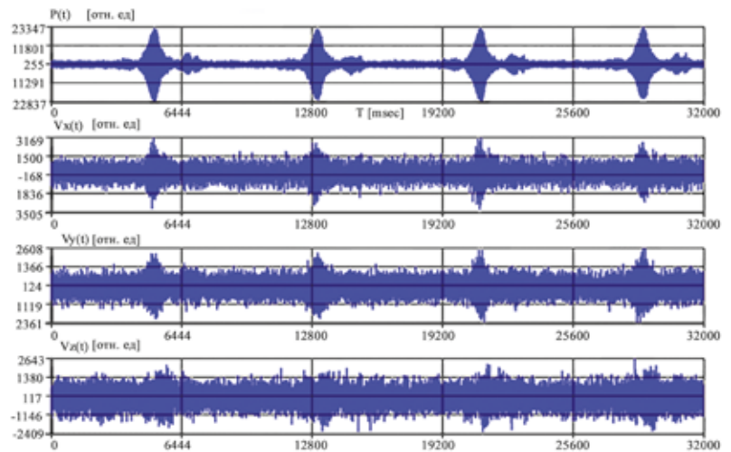
Рис. 13. Временная структура сигналов в каналах КП, приемный модуль ПМ-1
