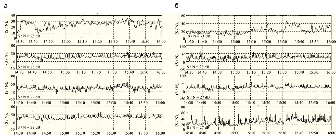
Рис. 11. Проходные характеристики для отношения (S/N) в каналах КП, приемные модули: ПМ-1 (а); ПМ-2 (б); ПМ-3 (в), частотный диапазон 16–20 Гц, время усреднения 50 с
