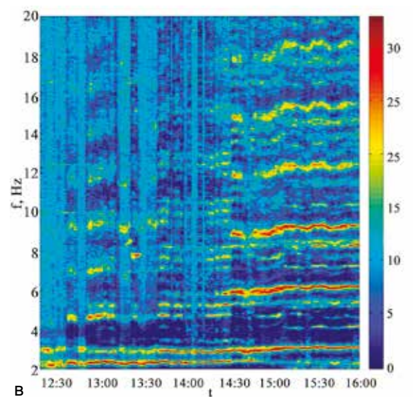
Рис. 9. Сонограммы на выходе БОС для отношения (S/N), приемные модули: ПМ-1(а); ПМ-2(б); ПМ-3 (в)
