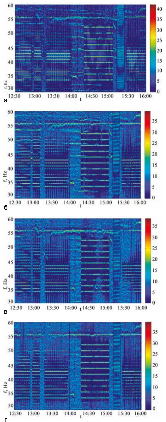
Рис. 7. Сонограммы для отношения (S/N) на выходе канала звукового давления (а) и в векторных каналах ( v_x , v_y , v_z ), (б, в, г), приемный модуль ПМ-1
