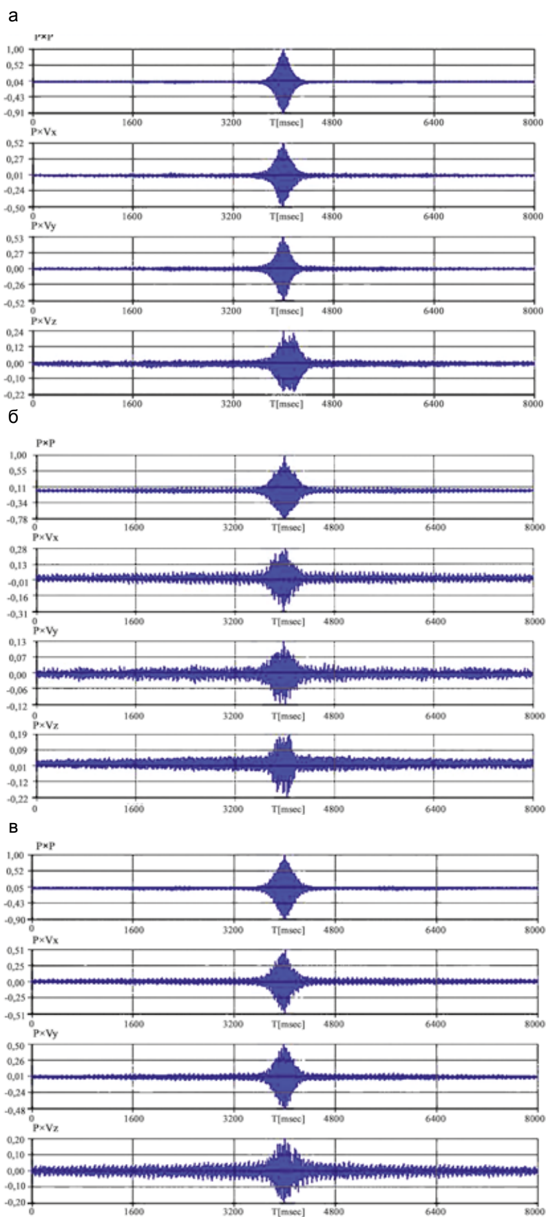
Рис. 17. Коэффициенты автокорреляции и взаимной корреляции в каналах КП, приемные модули: ПМ-1 (а); ПМ-2 (б); ПМ-3 (в);
