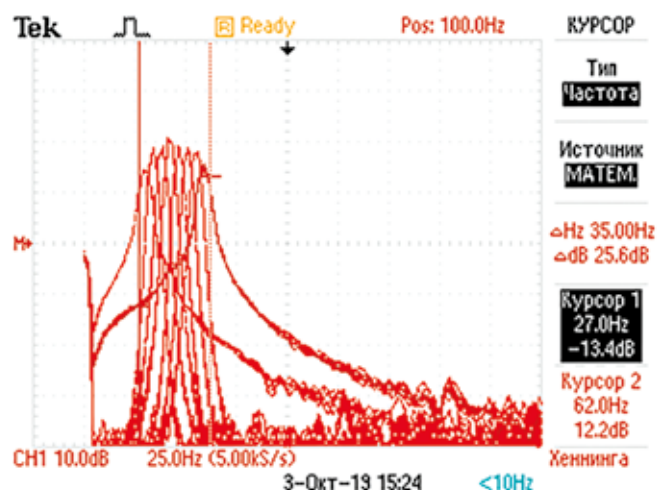
Рис. 4. Спектр ЛЧМ-сигнала в диапазоне частот 30–60 Гц
