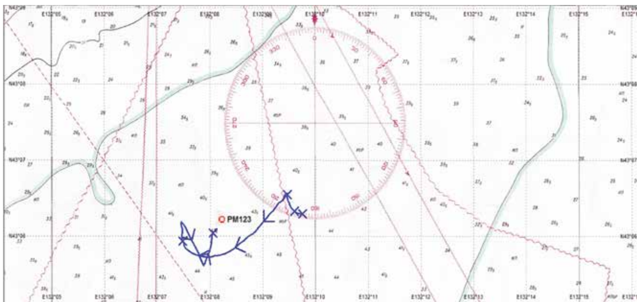
Рис. 2. Схема маневрирования НИС «Юрий Молоков» относительно приемных модулей ПМ-1, 2, 3
